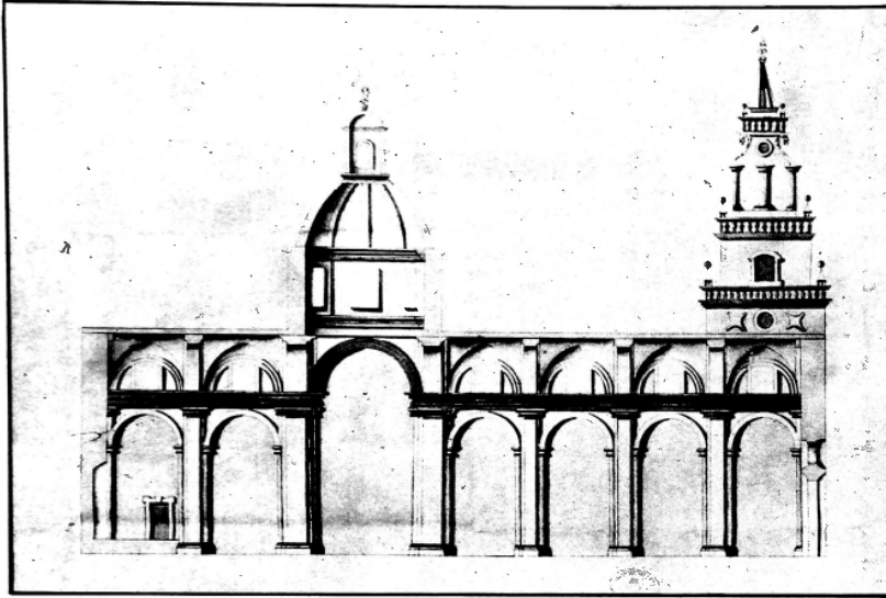
"Perfil por todo el Largo de la Yglesia", del proyecto presentado por Lazo de la Vega en 1735. Este proyecto para la Parroquia Mayor ha permanecido hasta ahora inédito y las fotografías que ahora publicamos constituyen reproducciones directas de los planos que se guardan en el Archivo de Indias.
